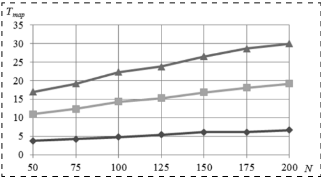
Рис. 3. Зависимость времени выбора лидера от числа роботов для K = 8
