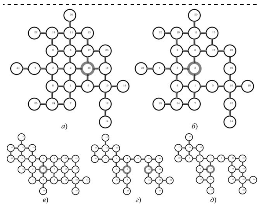
Рис. 1. Переголосование. Толстой линией выделен лидер
