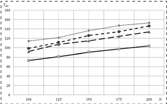
Рис. 7. Время кластеризации: сплошная линия — 4 кластера, длинная штриховая — 6 кластеров, короткая штриховая — 8 кластеров, пунктирная линия — 10 кластеров
