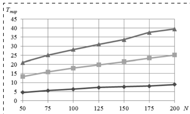
Рис. 2. Зависимость времени выбора лидера от числа роботов для K = 4
